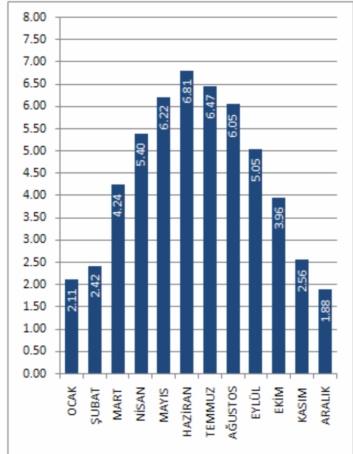
MUĞLA İLİ GLOBAL RADYASYON DEĞERLERİ (KWh/m 2 -gün)
